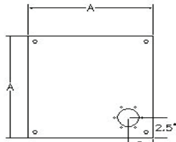
TVL-949 c/w Filler Cutout
